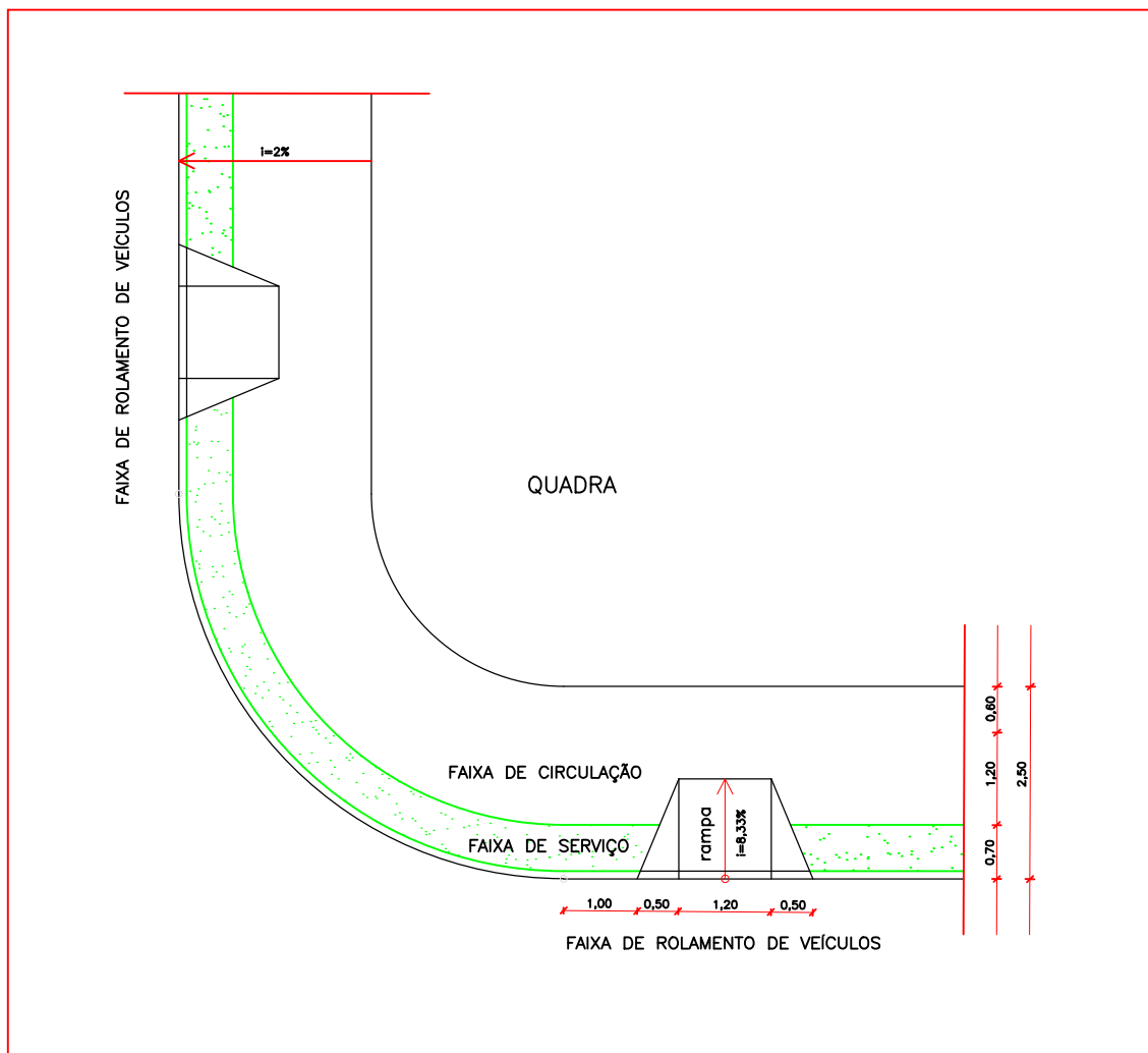
PLANTA - RAMPAS DE ESQUINA S/ESC
