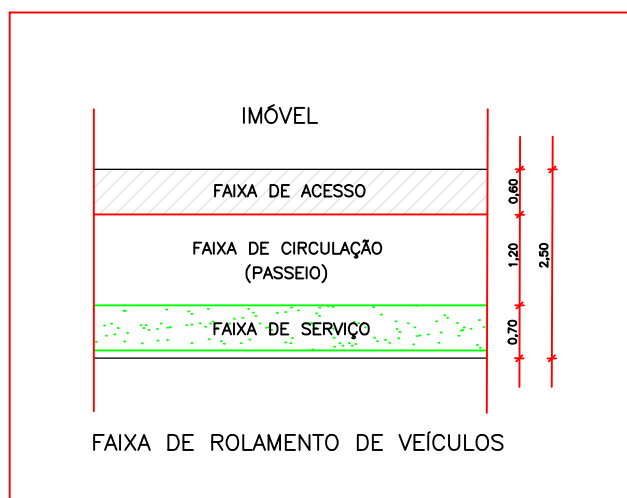
PLANTA - FAIXAS DA CALÇADA PÚBLICA S/ESC
